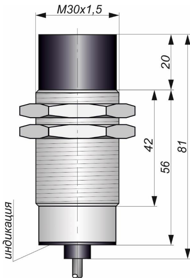
Габаритный чертеж
